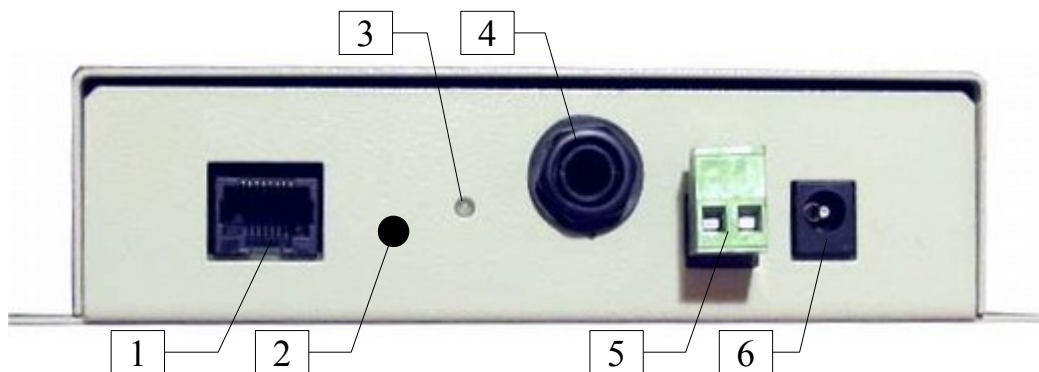
Рисунок 2.1 – Задняя панель ИТС-ЛС-О,
