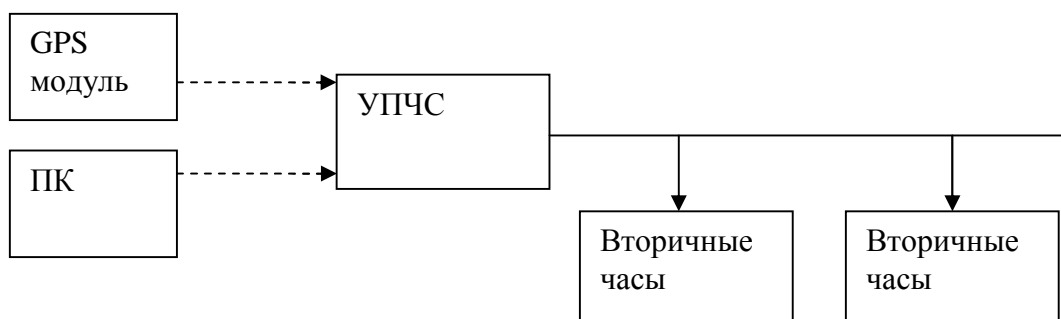
Рисунок 2.11 – Обобщенная схема часофикации
