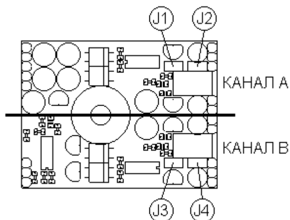
Рисунок III.4. Внешний вид платы расширения МП2(универсальная)
