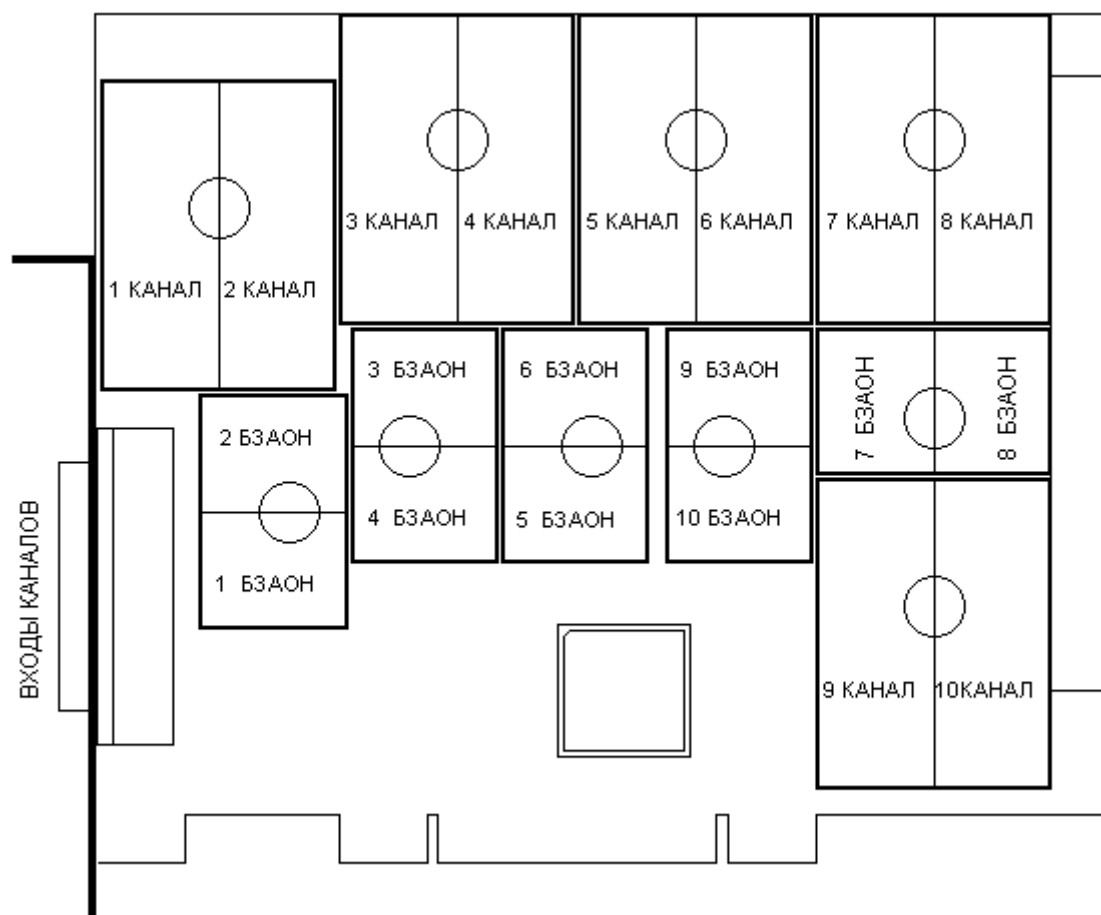
Рисунок III.2. Внешний вид кросс-платы МПМ-12 (PCI) и расположение
