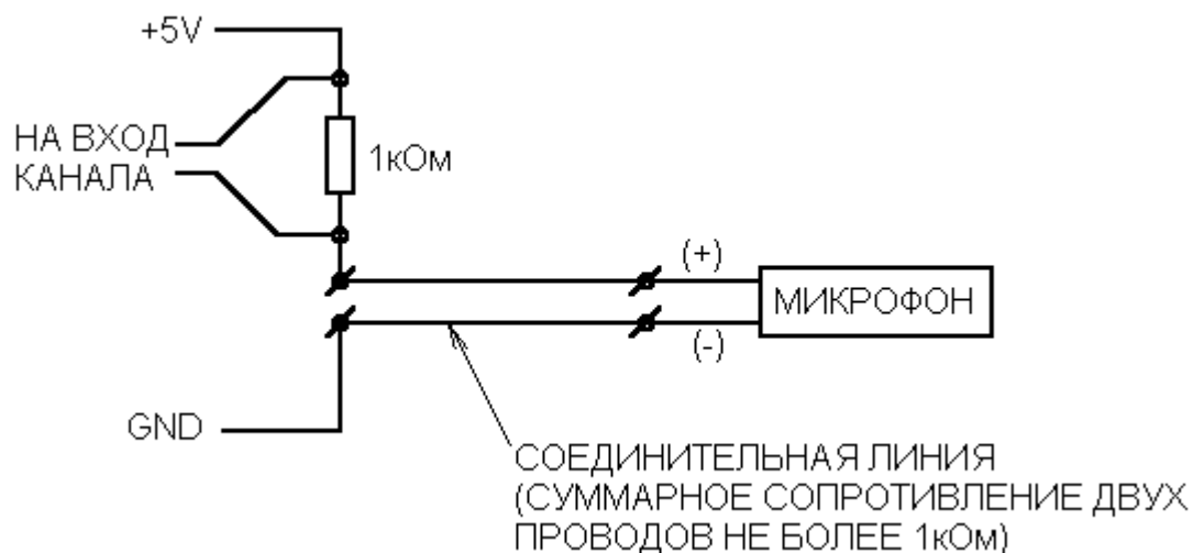
Рисунок III.5. Подключение активного микрофона
