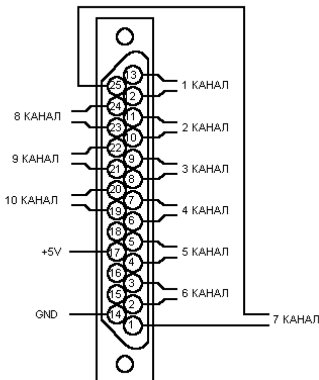
Рисунок III.3.Распайка входного разъема кросс-платы МПМ-12(USB)
